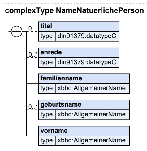
Abbildung II.4.9. NameNatuerlichePerson
