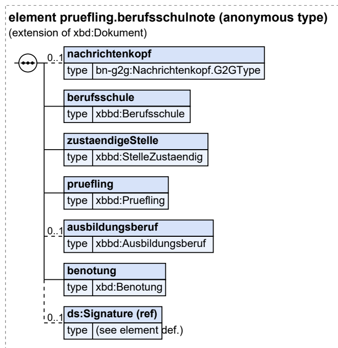
Abbildung II.6.5. pruefling.berufsschulnote
