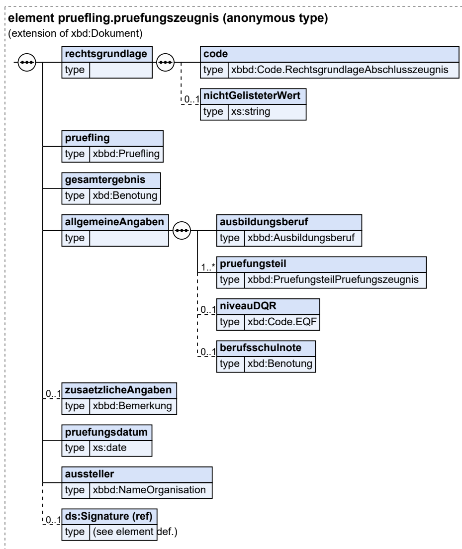
Abbildung II.6.1. pruefling.pruefungszeugnis
