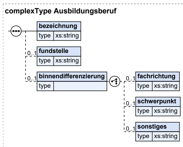
Abbildung II.5.2. Ausbildungsberuf
